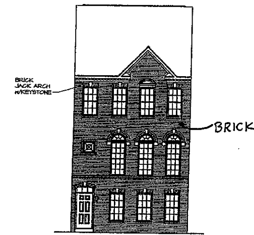
4 FRONT ELEVATION "C" SCALE: 1/8" = 1'-0"
