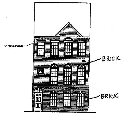
3 FRONT ELEVATION "C" SCALE: 1/8" = 1'-0"
