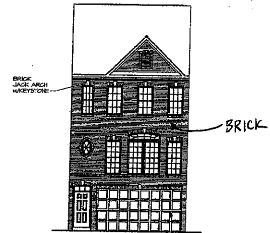
4 FRONT ELEVATION "D" SCALE: 1/8" = 1'-0"
