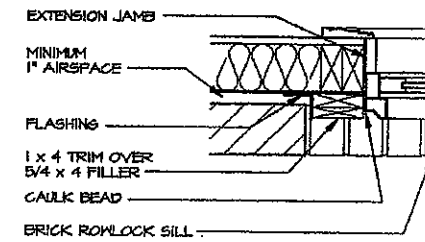
4 WINDOW TRIM SECTION SCALE: 1 1/2\" = 1'-0"
