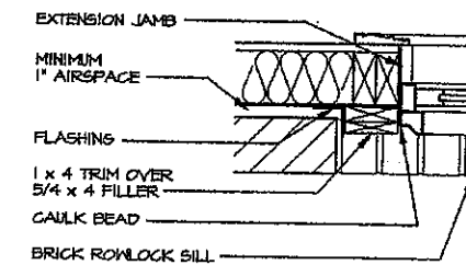
WINDOW TRIM SECTION SCALE: 1/2" = 1'-0"
