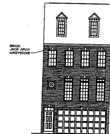
4 FRONT ELEVATION "A" SCALE: 1/8" = 1'-0"
