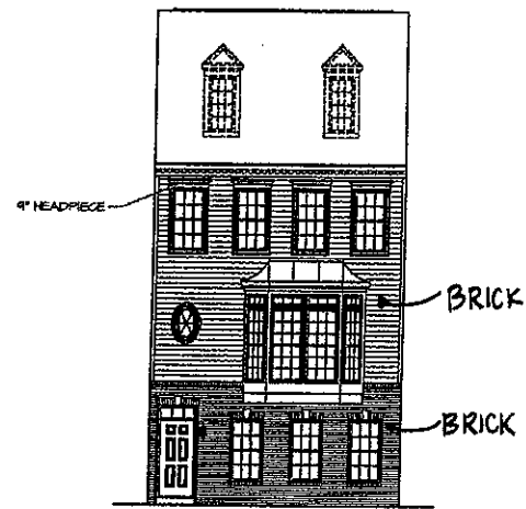
3 FRONT ELEVATION "E" SCALE: 1/8" = 1'-0"
