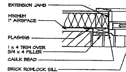
3 A-1 WINDOW TRIM SECTION SCALE: 1 1/2" = 1'-0"
