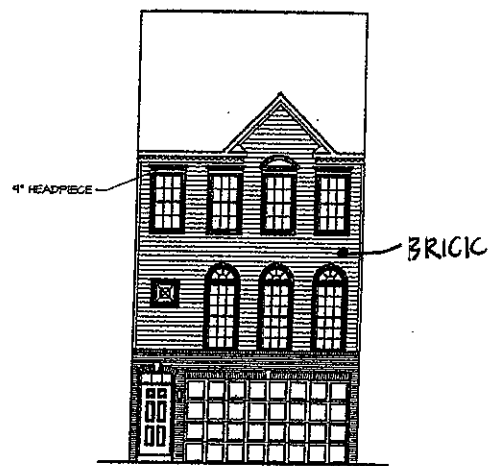
5 FRONT ELEVATION "C" SCALE: 1/8" = 1'-0"
