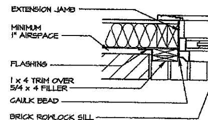
4 WINDOW TRIM SECTION SCALE: 1/2" = 1'-0"
